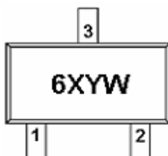
SOT-23-3L
