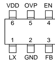
TSOT-23-6
