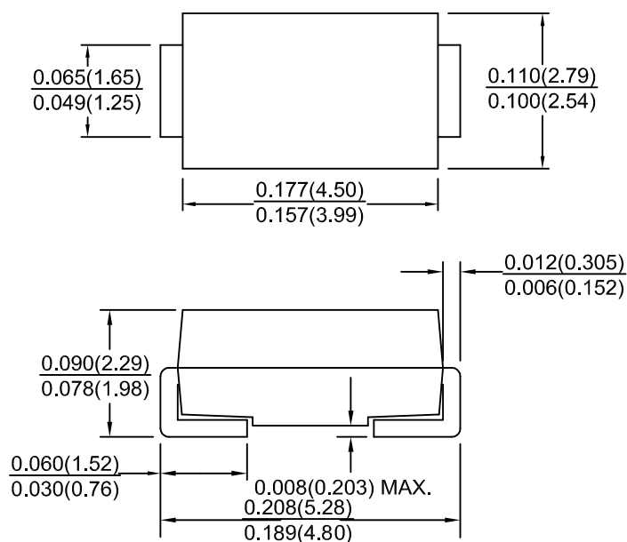
SMA/DO-214AC
