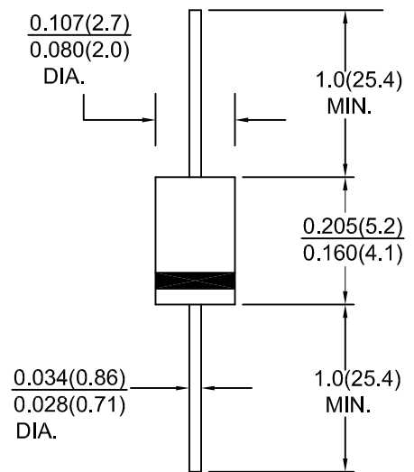
DO-204AL(DO-41)
